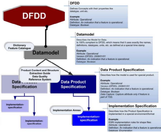
Şekil-8. DFDD Veri Modeli ve Hiyerarşisi
