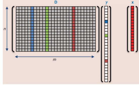
Şekil 1. Seyreklik modeli. Model \mathbf{D}\gamma = x olacak şekilde x işaretini modeller (Pappyan vd., 2018).
