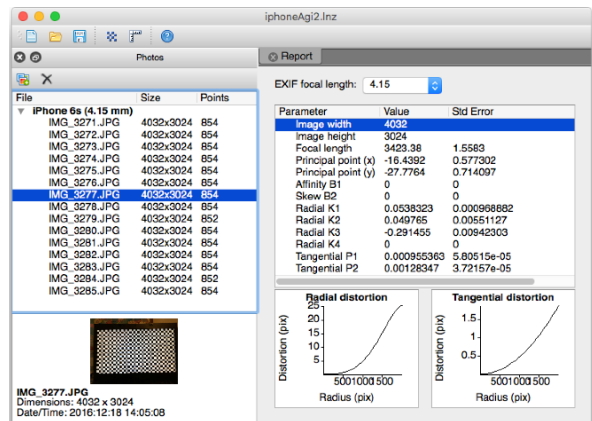
Şekil 9. Agisoft Lens grafik ara yüzü
