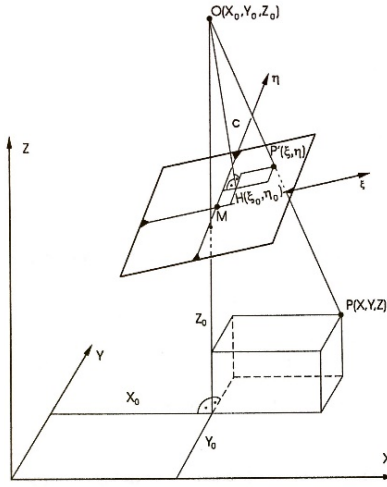
Şekil 1. Kolinearite koşulu, resim ve cisim koordinatları
