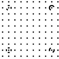
Şekil 6. PMS kalibrasyon test alanı (A4)
