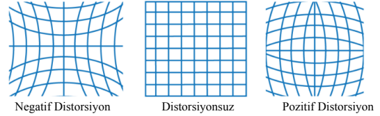
Şekil 2. Radyal distorsiyonun görüntüye etkileri (MathWorks, 2017a)
